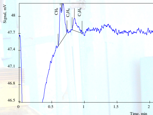
Хроматограмма углеводородов в аммиаке
