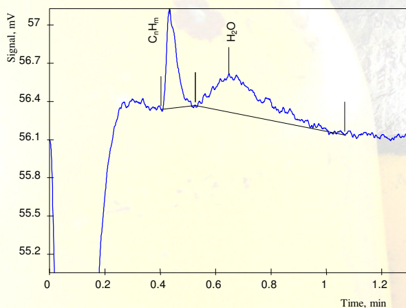
Хроматограмма общего углерода и воды в аммиаке
