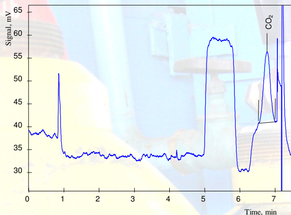
Хроматограмма диоксида углерода в аммиаке
