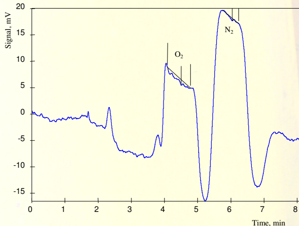
Хроматограмма азота и кислорода в аммиаке
