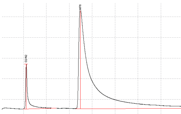
Хроматограмма гексафторида вольфрама
