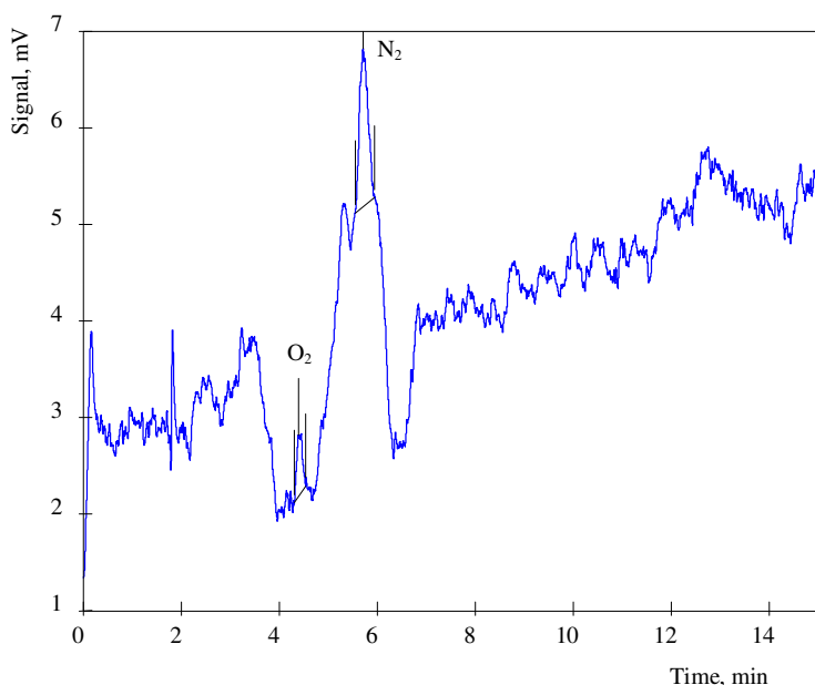
Хроматограмма водорода, кислорода, азота и оксидов углерода в моногермана
