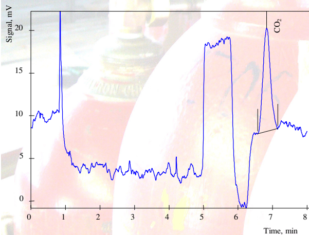
Хроматограмма диоксида углерода в моносилане
