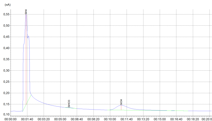
Хроматограмма хлорорганических соединений и хлорсиланов в моносилане
