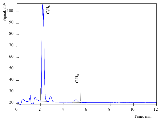
Хроматограмма углеводородов в моносилане
