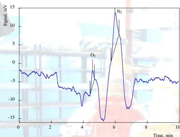
Хроматограмма кислорода и азота в моносилане
