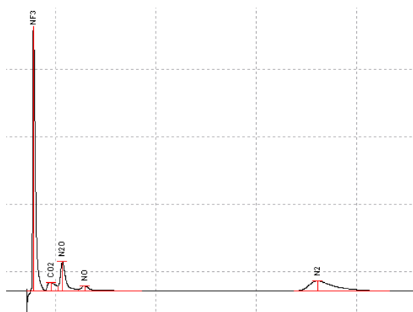
Хроматограмма трифторида азота (синтез-газ)
