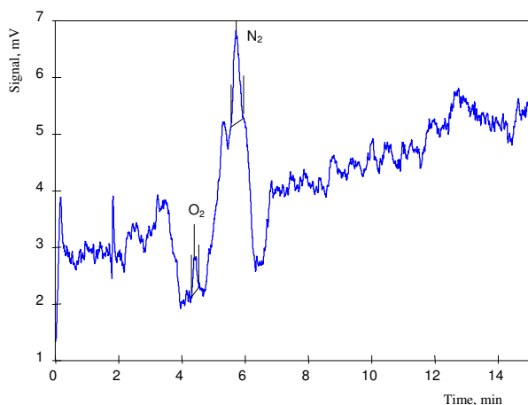
Хроматограмма водорода, кислорода, азота и диоксида углерода в трифториде азота (концентрации водорода и диоксида углерода ниже предела обнаружения)
