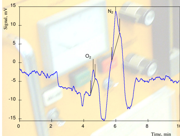
Хроматограмма азота и кислорода в закиси азота
