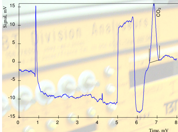
Хроматограмма диоксида углерода в закиси азота
